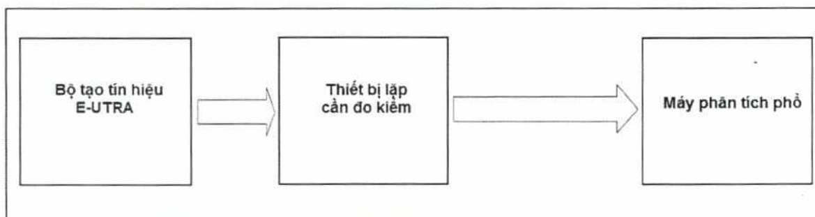
Hình C. 3 – Sơ đồ đo phát xạ không mong muốn: Phát xạ không mong muốn băng tần hoạt động
